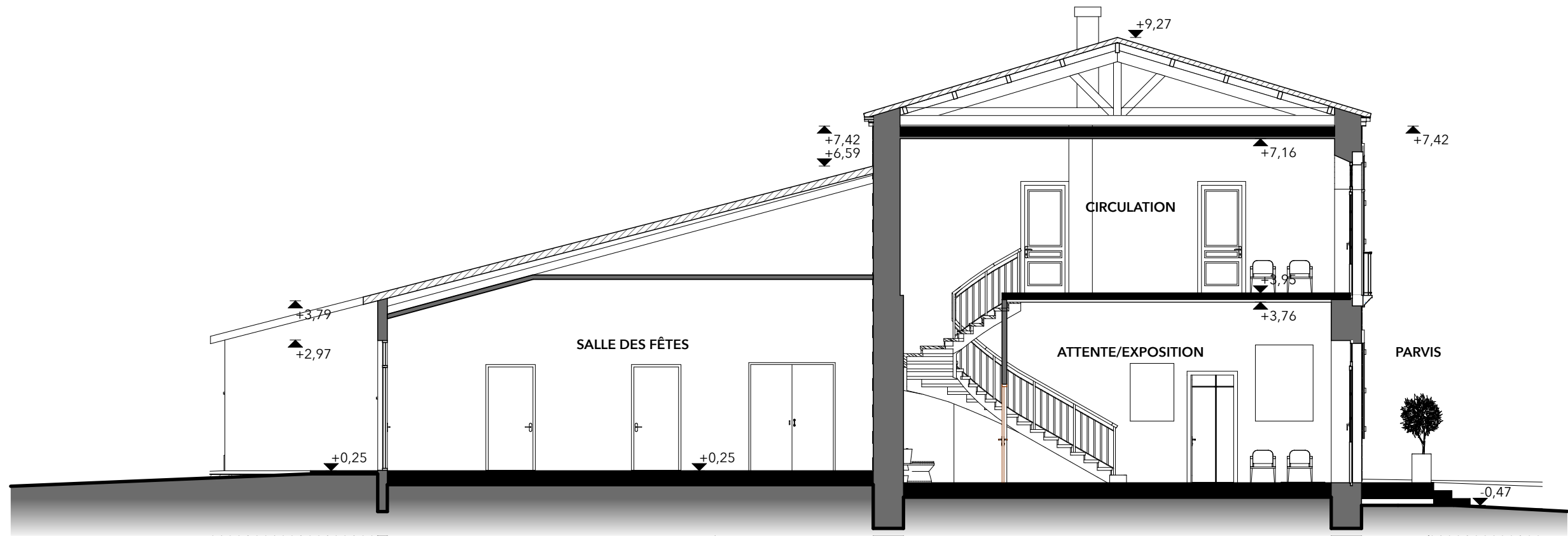
COUPE C
