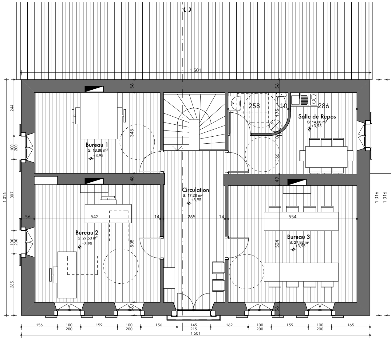
PLAN NIVEAU 2
